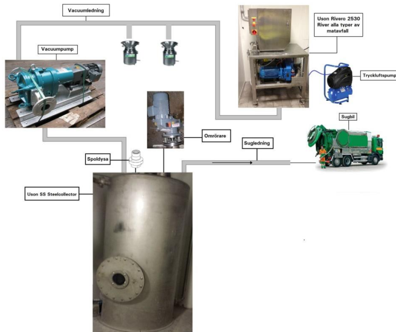
Uson Rivero 2530 - Vacuumsystem
